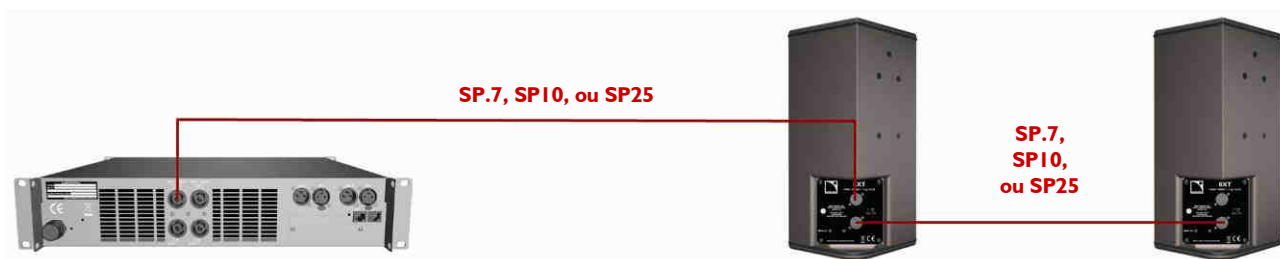
Figure 4 : Raccordement de deux 8XT en parallèle sur le canal I du LA4 / LA4X
